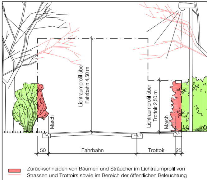
Abbildung 3, Lichtraumprofil Strasse
